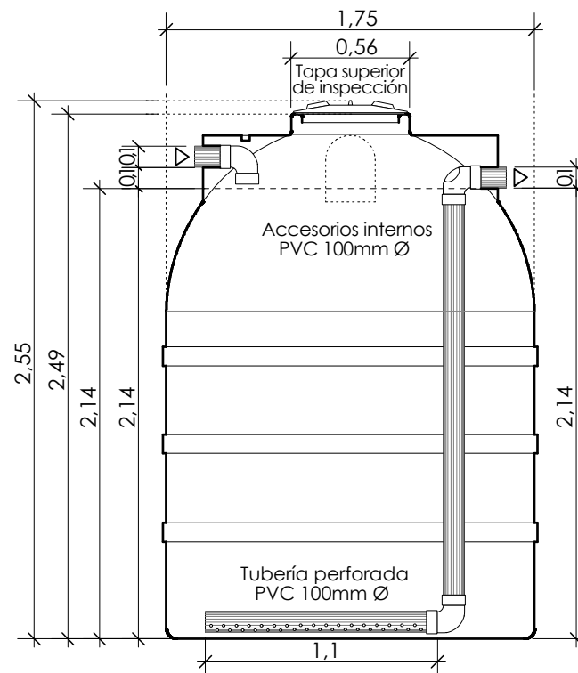
SECCIÓN TRANSVERSAL
