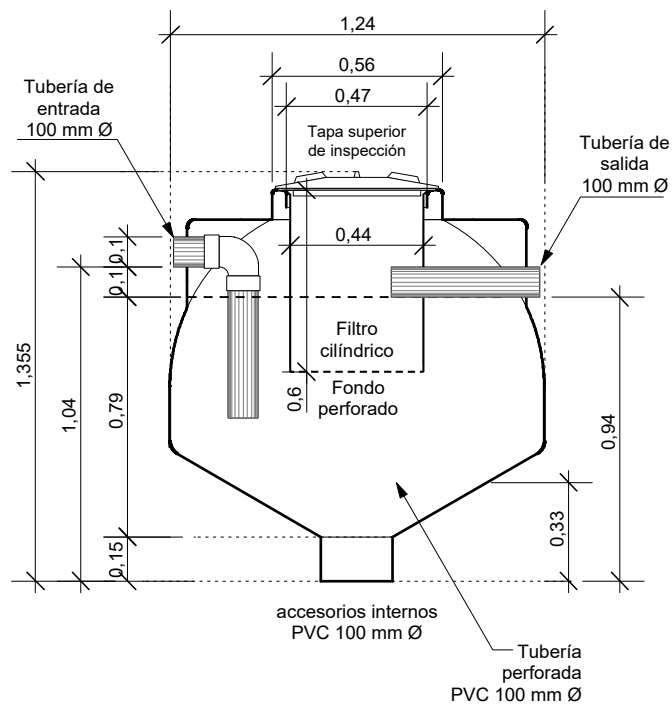
sección transversal A
