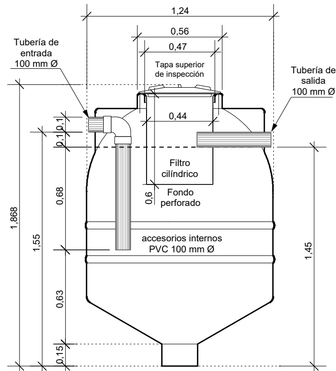
sección transversal A escala 1:25
