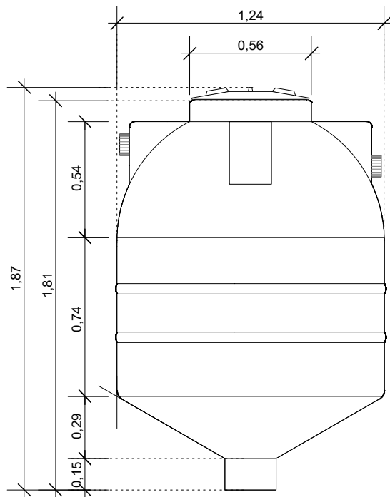
vista lateral escala 1:25
