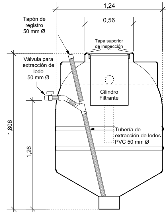
sección transversal B escala 1:25
